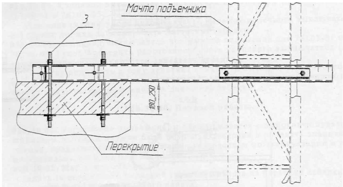
Рис 3А Схема установки опоры настенной верхней для ПМГ-1-Б-76103-03
